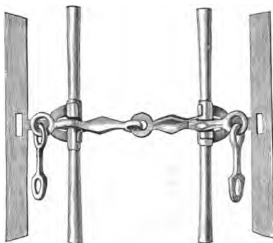
573—576. Bidselmundbid af Jern. Mors de bride en fer.
